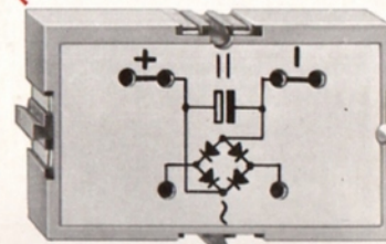
1 Gleichrichter-Baustein
